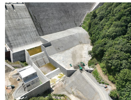
減勢工下流 【ICT施工技術による見事な整形】 2026年8月18日 撮影
